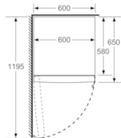
Dimensiones en mm
