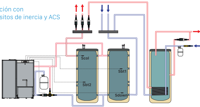
Instalación con 2 depósitos de inercia y retorno invertido
